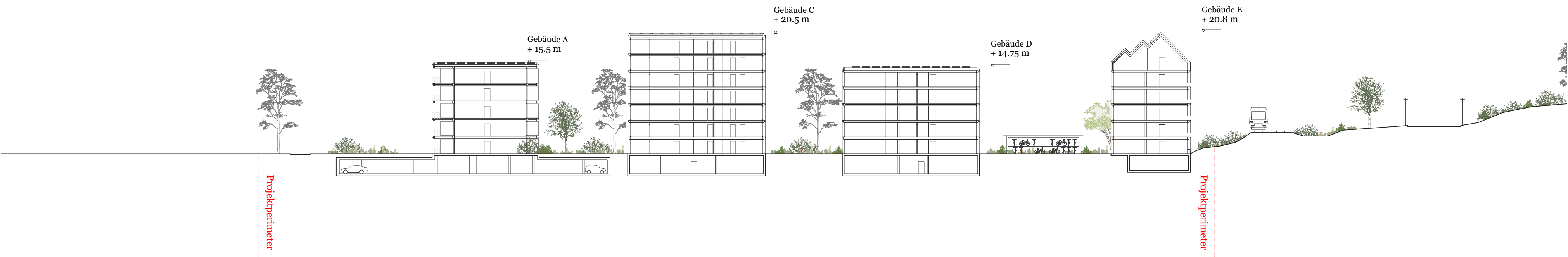
Schnitt BB 1:500
