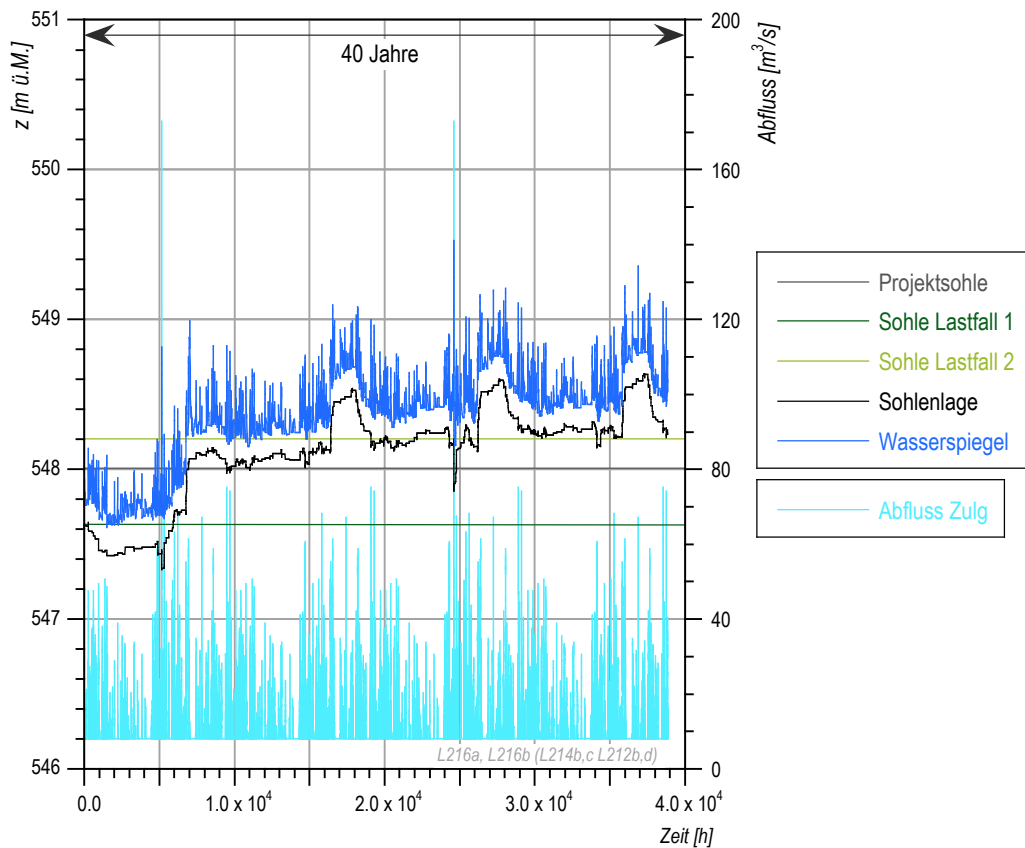
Abbildung 16: Entwicklung der Sohlenlage in der Aufweitung, Referenzquerschnitt km 0.247. Die tiefe Sohle in den ersten 10'000 h entspricht dem Modelleffekt, dass Geschiebe von Oberlauf Zeit braucht, um in die Aufweitung zu kommen. Diese Situation kann in der Realität z.B. kommen, wenn Geschiebe in einem grossen Ereignis im Schwemmholtzrechen zurückgehalten wird. Für die Herleitung der Abflussganglinien siehe 6.2.4.
