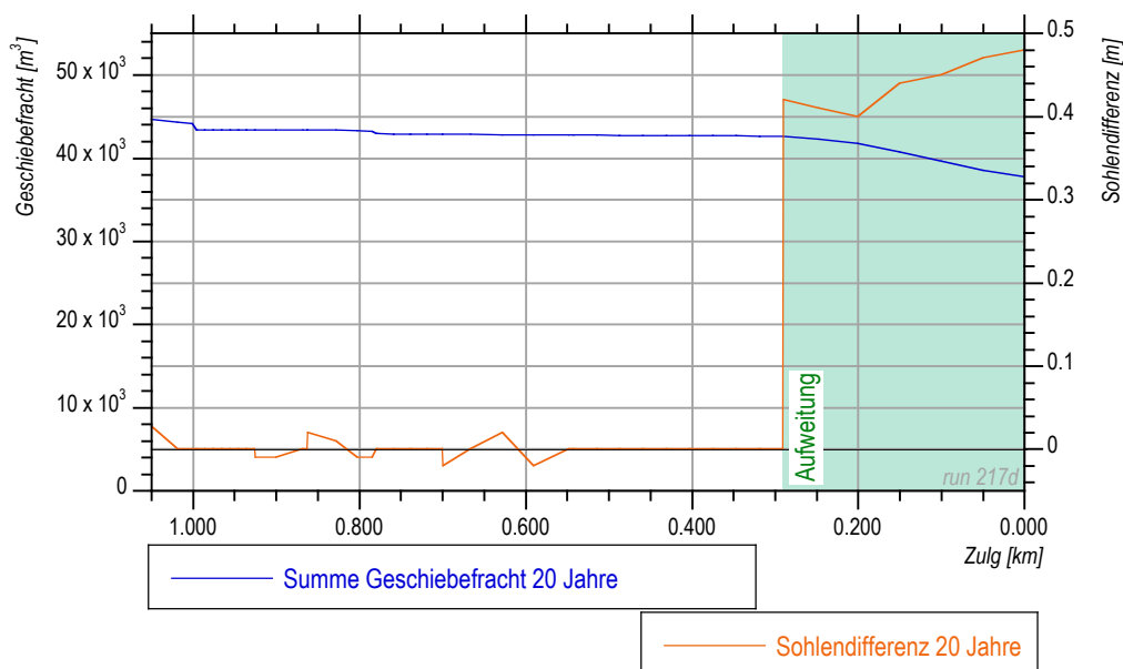
Abbildung 12: Geschiebefracht und Sohlendifferenz über 20 Jahre Modellierung.
