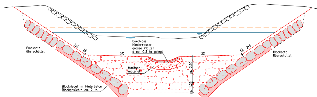
Abbildung 13: Schema Traversensystem mit Fischschlitz (1:250) aus [2].
