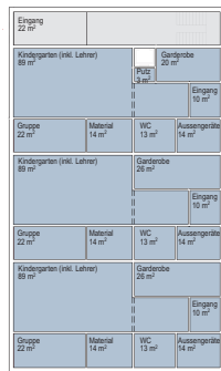
Abb. 3 Grundrisse Erdgeschoss, 1. und 2. Obergeschoss
