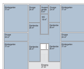
Abb. 6 Grundrisse Erdgeschoss und 1./2. Obergeschoss
