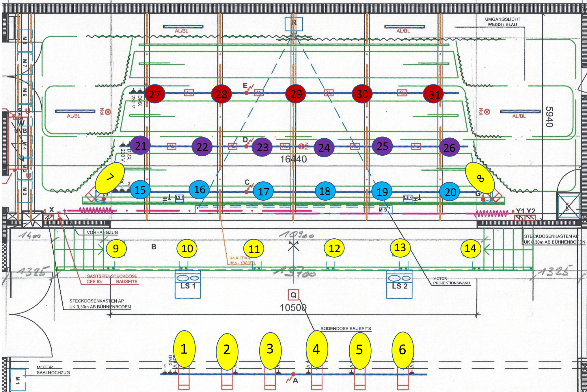
AULA Heimberg, Scheinwerferarchitektur
